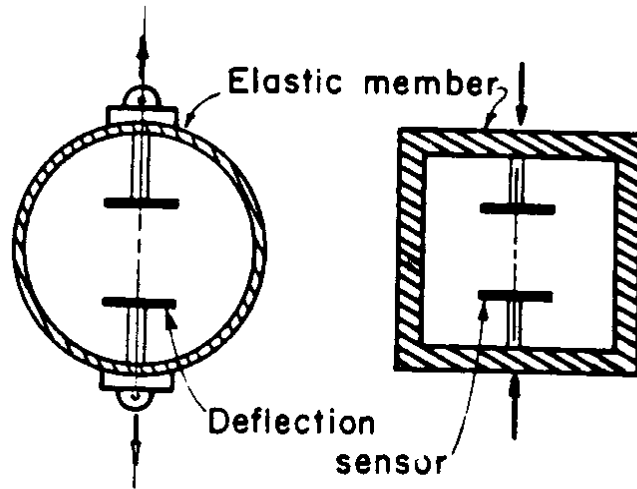
b) Load cells
