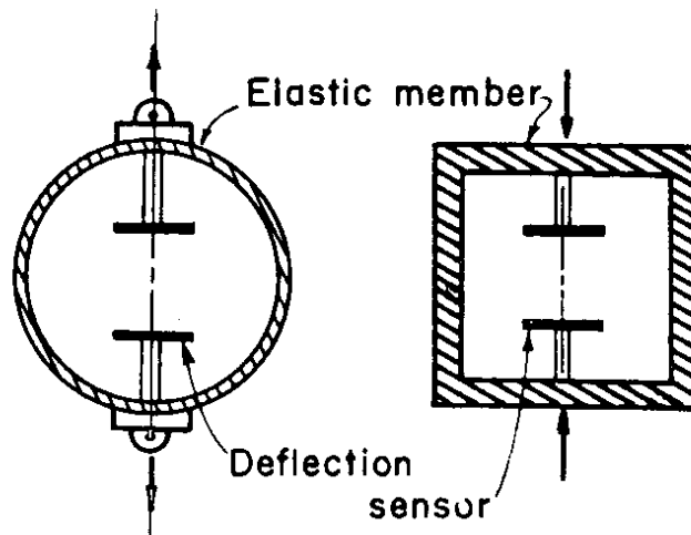
b) Load cells
