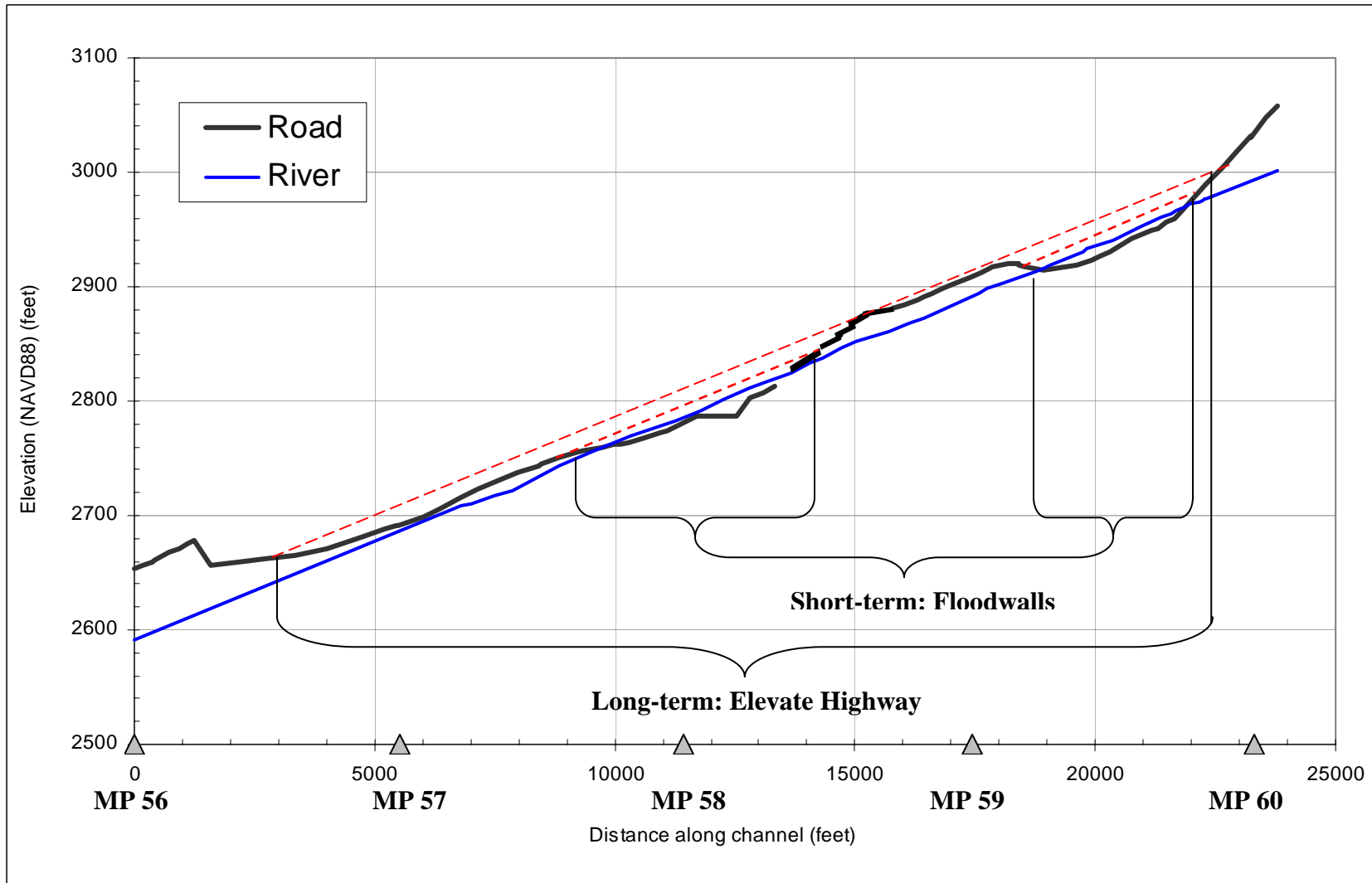
Figure D-2. Longitudinal Profile.
